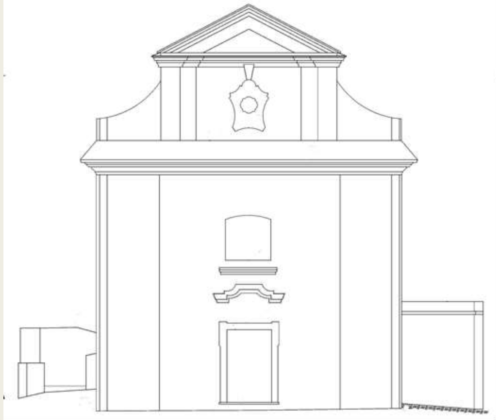
Obrázek 7 - Západní průčelí (2011)
