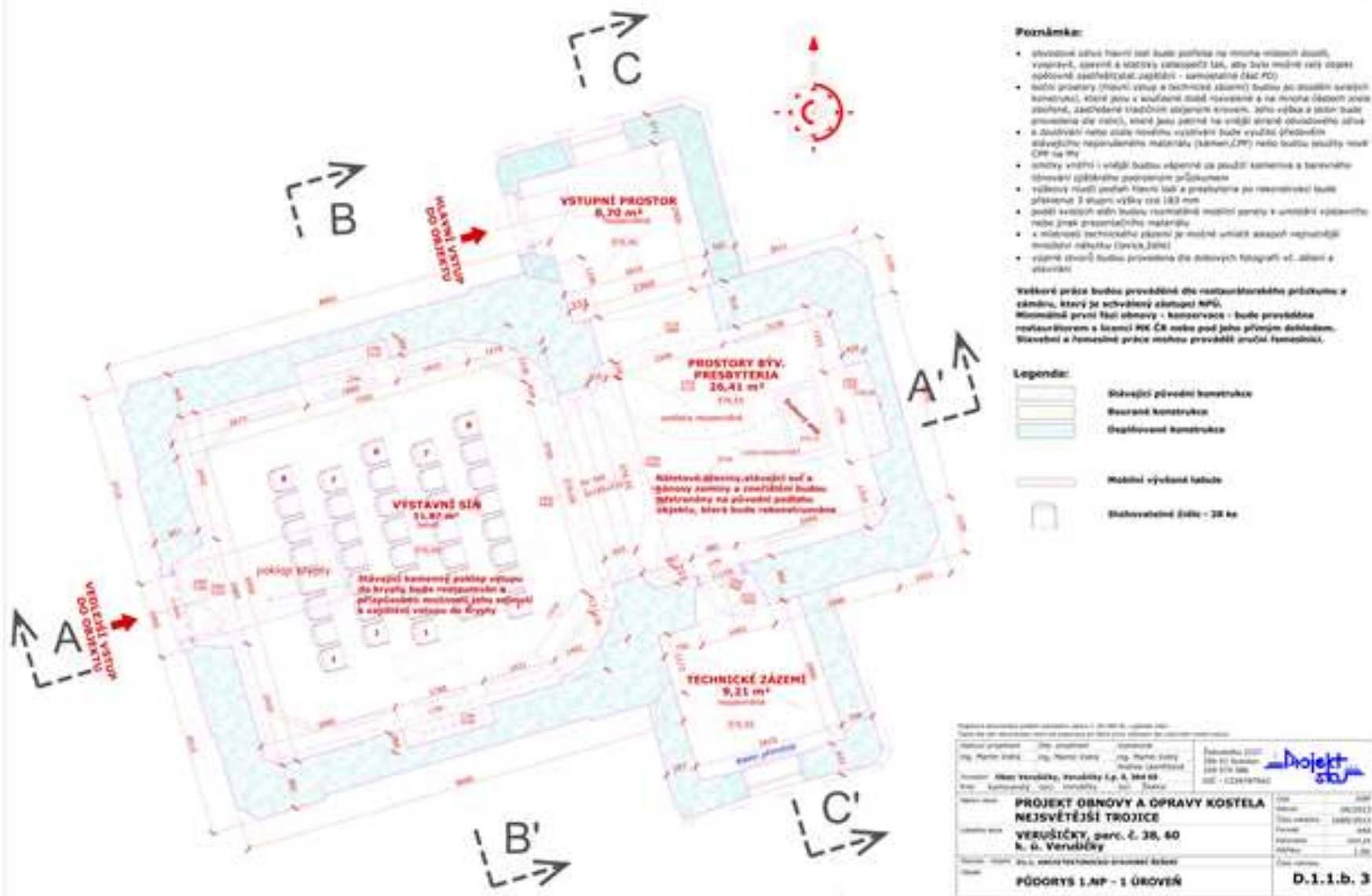
Obrázek 19 - PD - půdorys 1.NP
